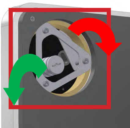
Abb. 1: Einstellung des Antiskating
