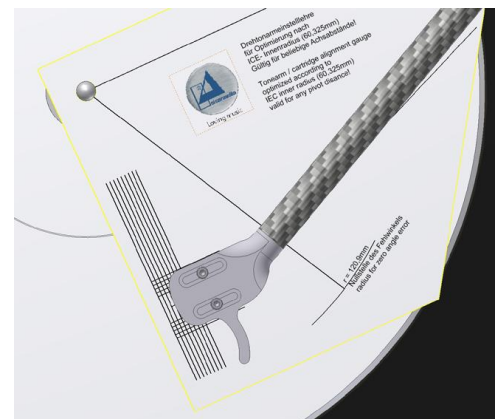
Abb 9: Parallelität des Tonarms
